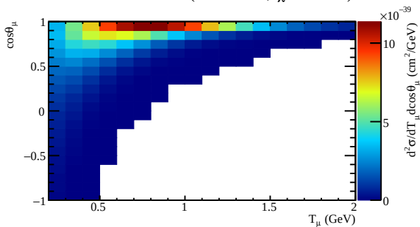
GENIE 2.12.0 ( \sigma=2.35\text{E-}37 , \chi^2=32341.0 )
