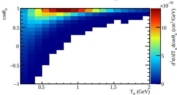
NEUT 5.3.6 ( \sigma=3.00\text{E-}37 , \chi^2=36894.0 )
