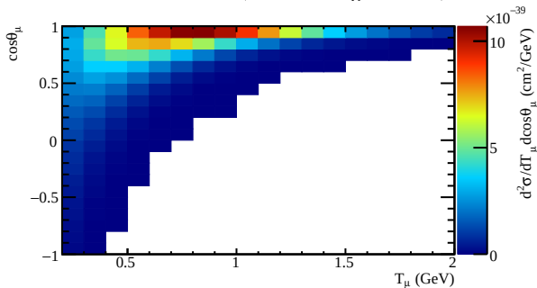
NUWRO v12 ( \sigma=2.46\text{E-}37 , \chi^2=35841.0 )
