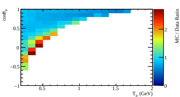
GENIE 2.12.0 / Data Ratio
